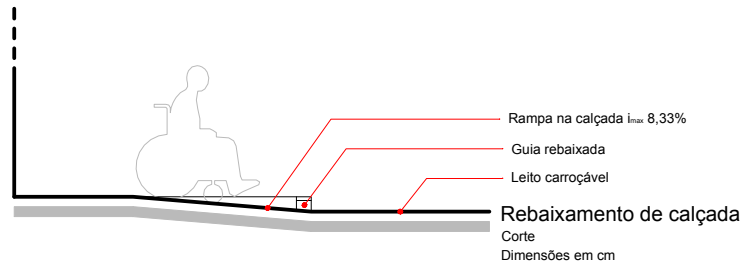
FIGURA 95 - PAG 79 NBR 9050 REBAIXAMENTO DE CALÇADA
