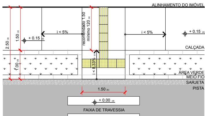
FIGURA 96 - PAG 81 NBR 9050 REBAIXAMENTOS DE CALÇADA ENTRE CANTEIROS
