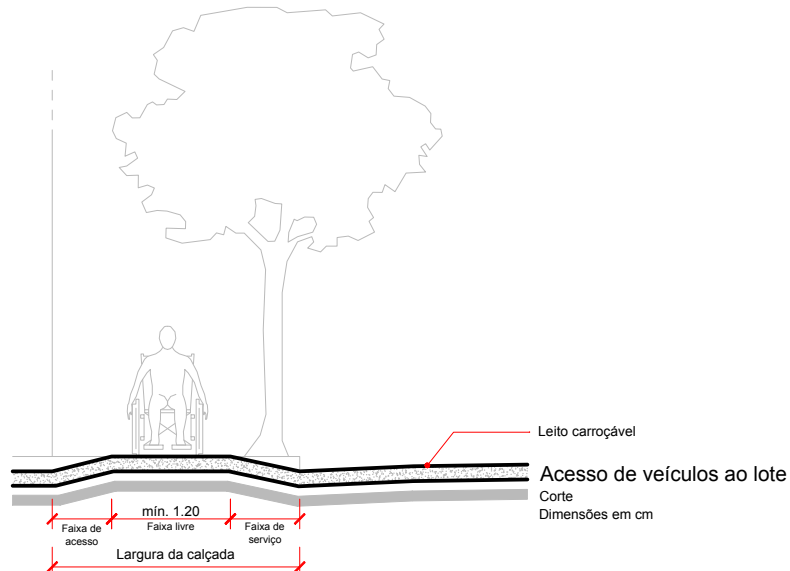
FIGURA 91 - PAG 78 NBR 9050 ACESSO DE VEÍCULOS AO LOTE
