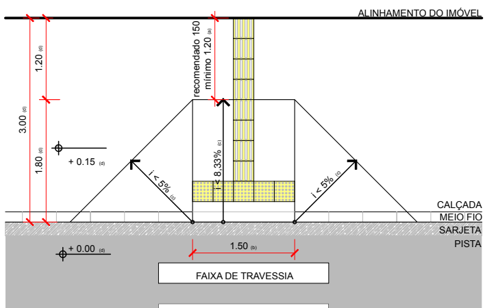
FIGURA 94 - PAG 79 NBR 9050 REBAIXAMENTO DE CALÇADA
