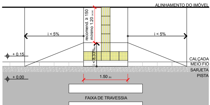
FIGURA 97 - PAG 81- NBR 9050 REBAIXAMENTOS DE CALÇADA ESTREITA
