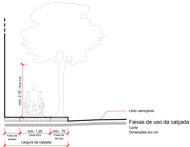
FIGURA 90 - PAG 75 NBR 9050 FAIXAS DE USO DA CALÇADA - CORTE
